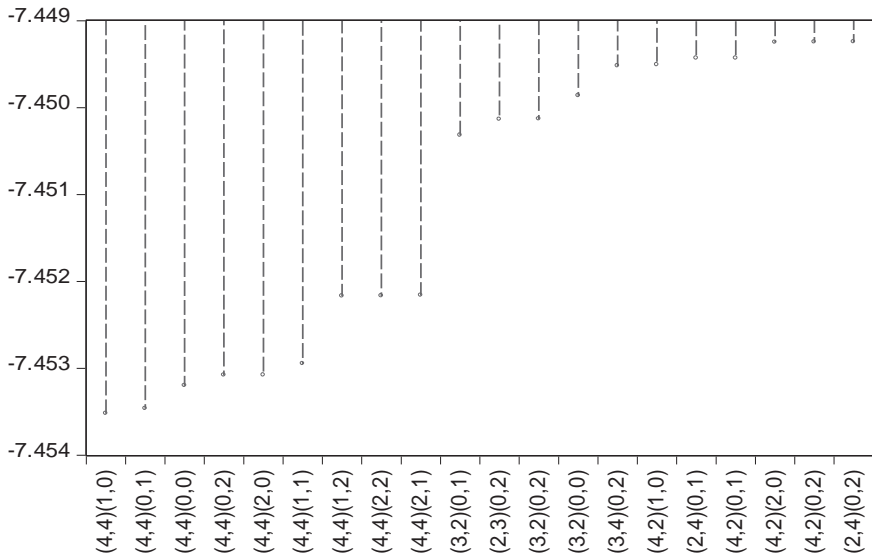
Gráfica de información del Criterio Akaike de los 20 mejores modelos. Akaike Information Criteria (top 20 models)
