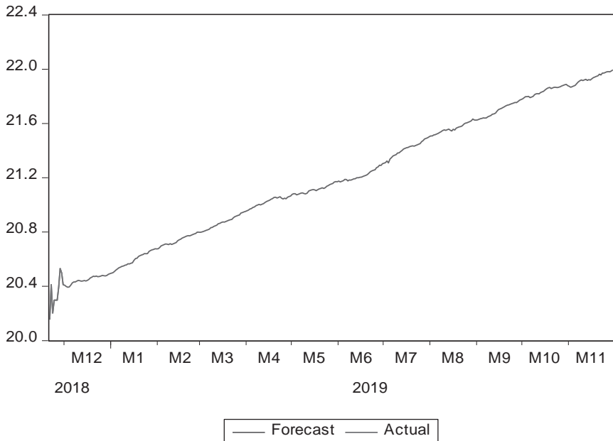
Gráfica del pronóstico del tipo de cambio a un año. Actual and Forecast
